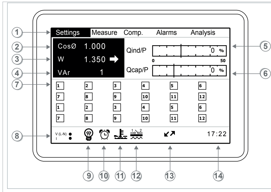
Figura 1.2: PFW03-M24
